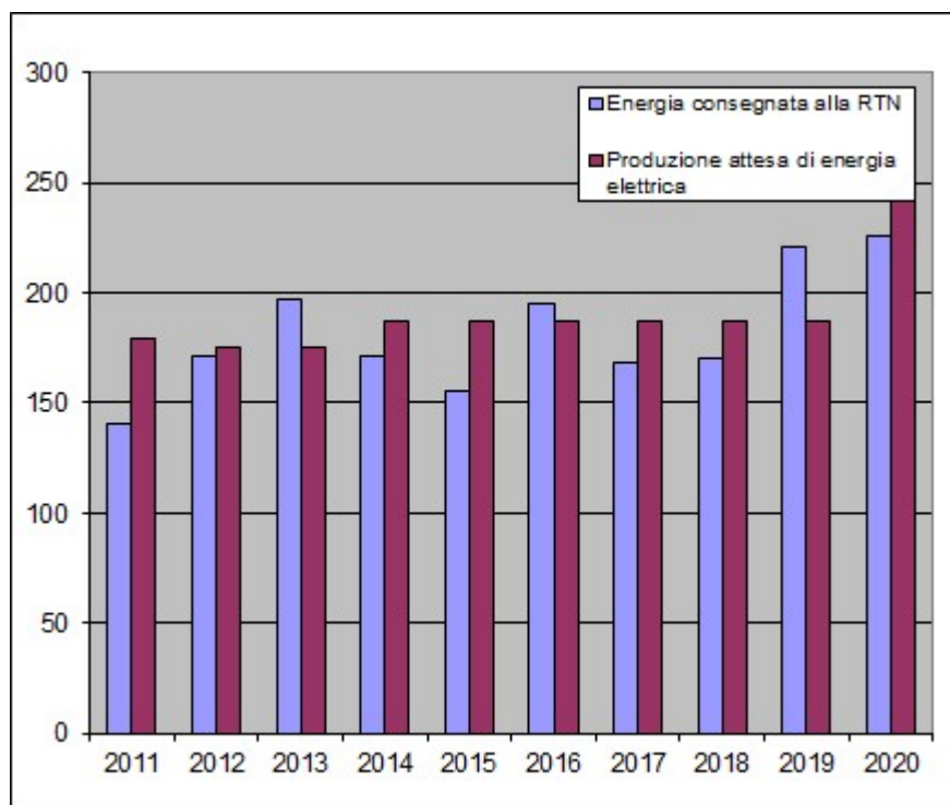
Figura 11: Energia consegnata vs produzione attesa
