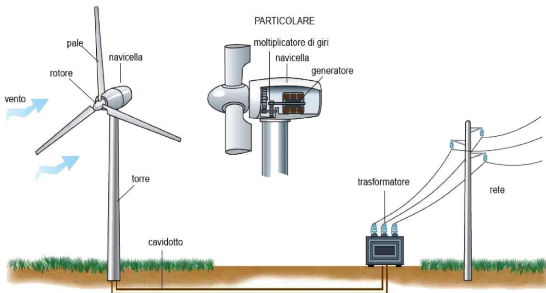
Figura 5. Schema di un impianto eolico
